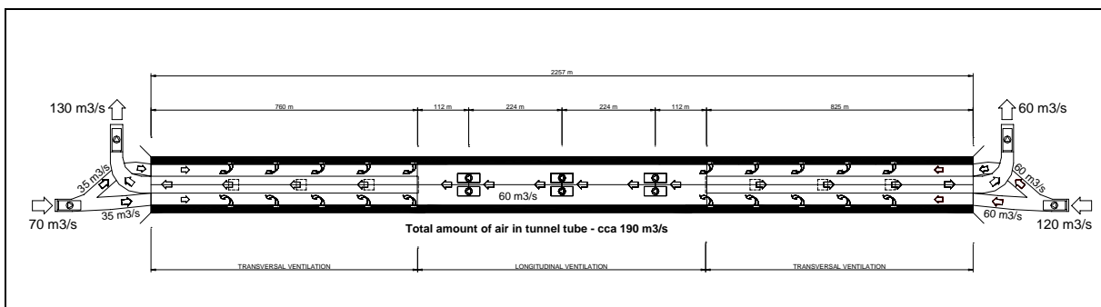
SCHEMA VĚTRÁNÍ
